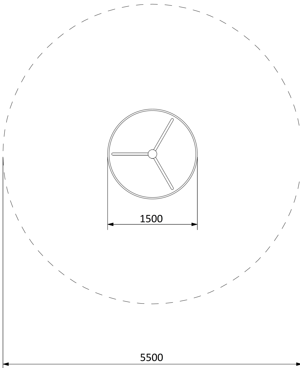
Rys. 1. Wymiary urządzenia i strefy bezpieczeństwa
