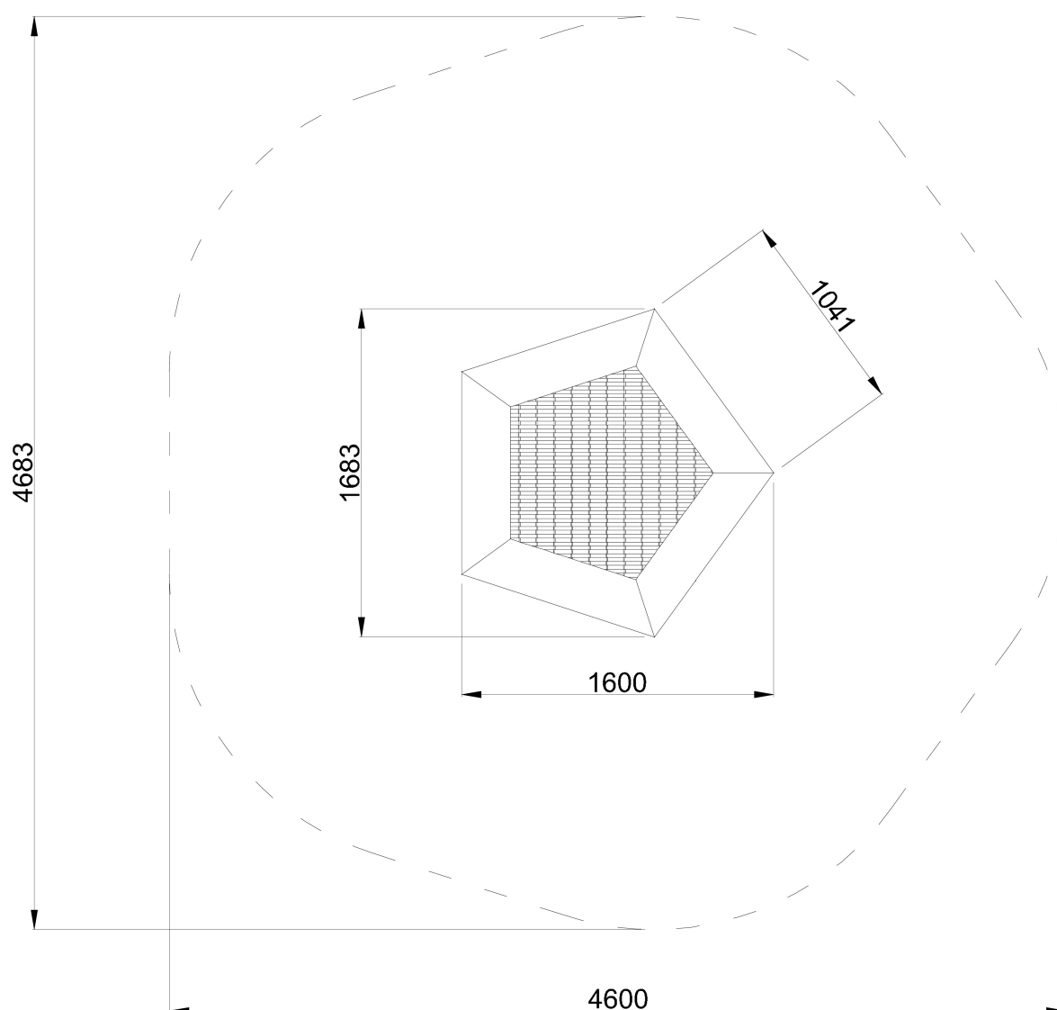
Rys. 1. Wymiary urządzenia i strefy bezpieczeństwa
