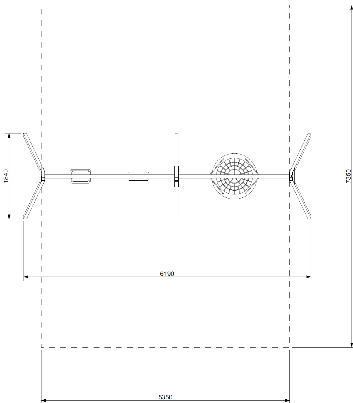
Rys. 1. Wymiary urządzenia i strefy bezpieczeństwa
